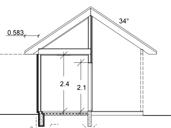
SNITT C-C
