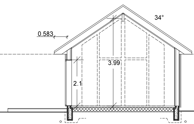
SNITT B-B
