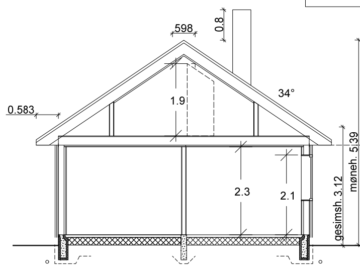
SNITT A-A
